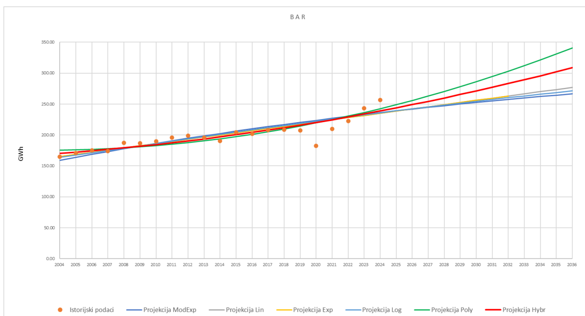
Slika 6-22. Grafički prikaz rezultata prognoznih modela za ED pogon Bar
