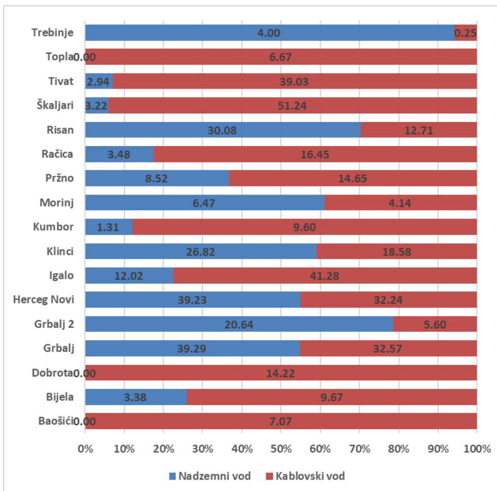
Slika 4-36 Učešće nadzemne i kablovske 10 kV mreže po napojnim TS Regiona 5
