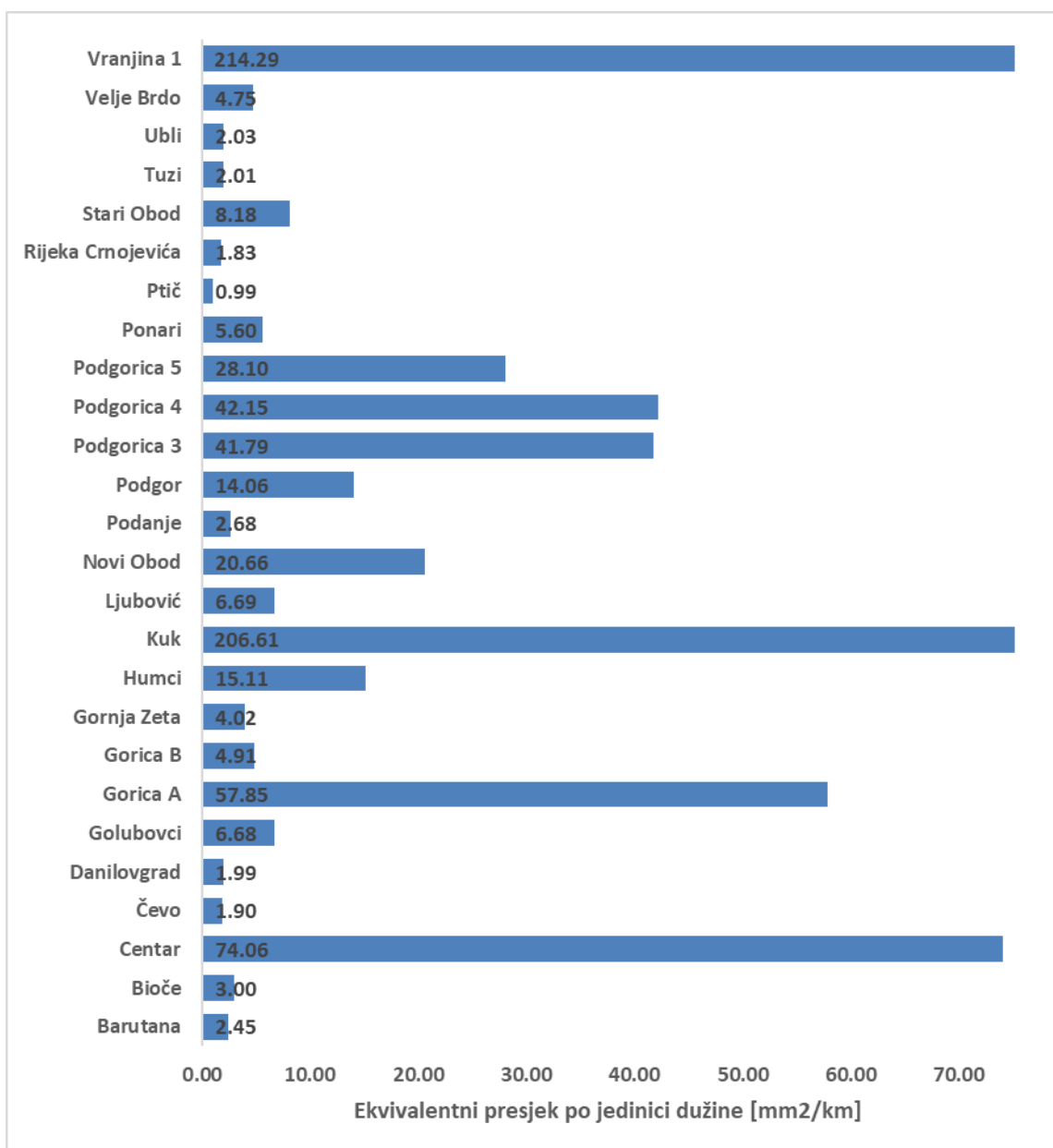
Slika 4-23 Ekvivalentni presjek po jedinici dužine (odnos ekvivalentnog presjeka i ekvivalentne dužine) 10 kV voda po napojnim TS Regiona 2 21
