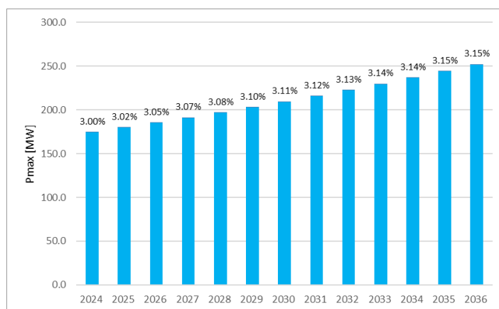
Slika 6-24. Prognoza vršnog opterećenja Regiona 4 za period 2024 – 2036. godina
