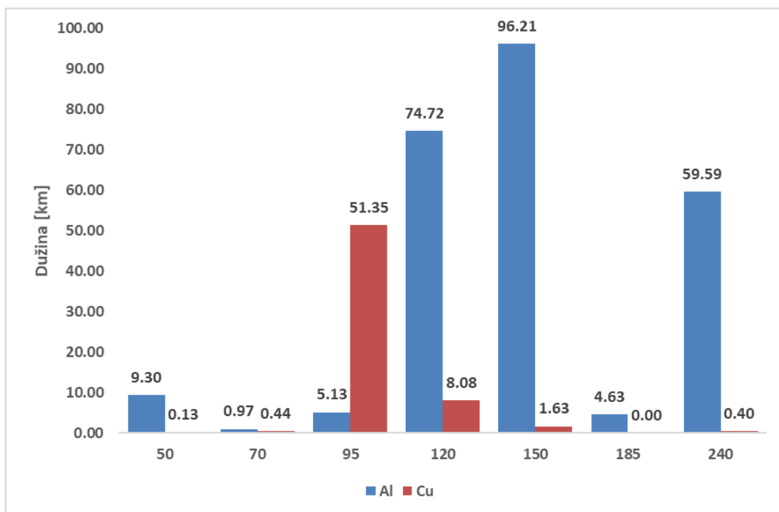
Slika 4-38 Struktura 10 kV kablovske mreže Regiona 5 prema presjecima [km]
