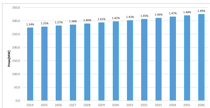
Slika 6-10. Prognoza vršnog opterećenja Regiona 2 za period 2024 – 2036. godina
