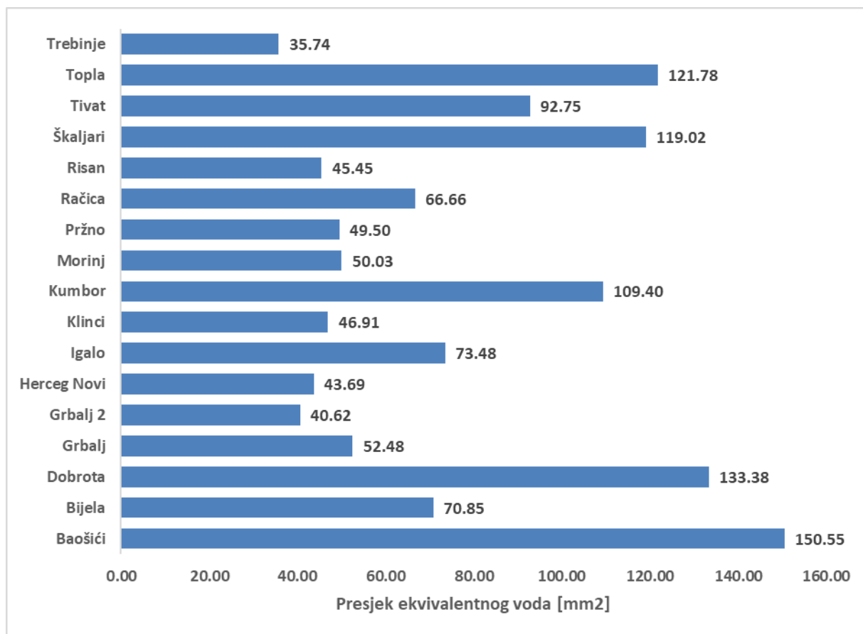
Slika 4-39 Presjek ekvivalentnog 10 kV voda po napojnim TS Regiona 5
