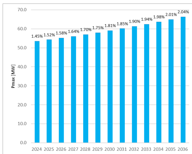
Slika 6-38. Prognoza vršnog opterećenja Regiona 6 za period 2024 – 2036. godina
