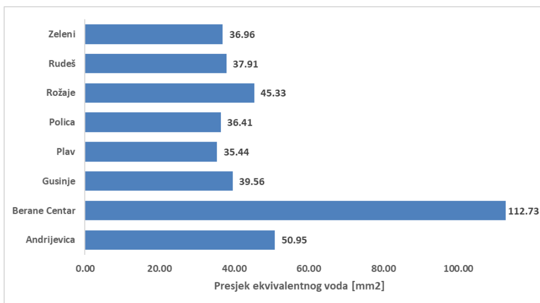
Slika 4-27 Presjek ekvivalentnog 10 kV voda po napojnim TS Regiona 3
