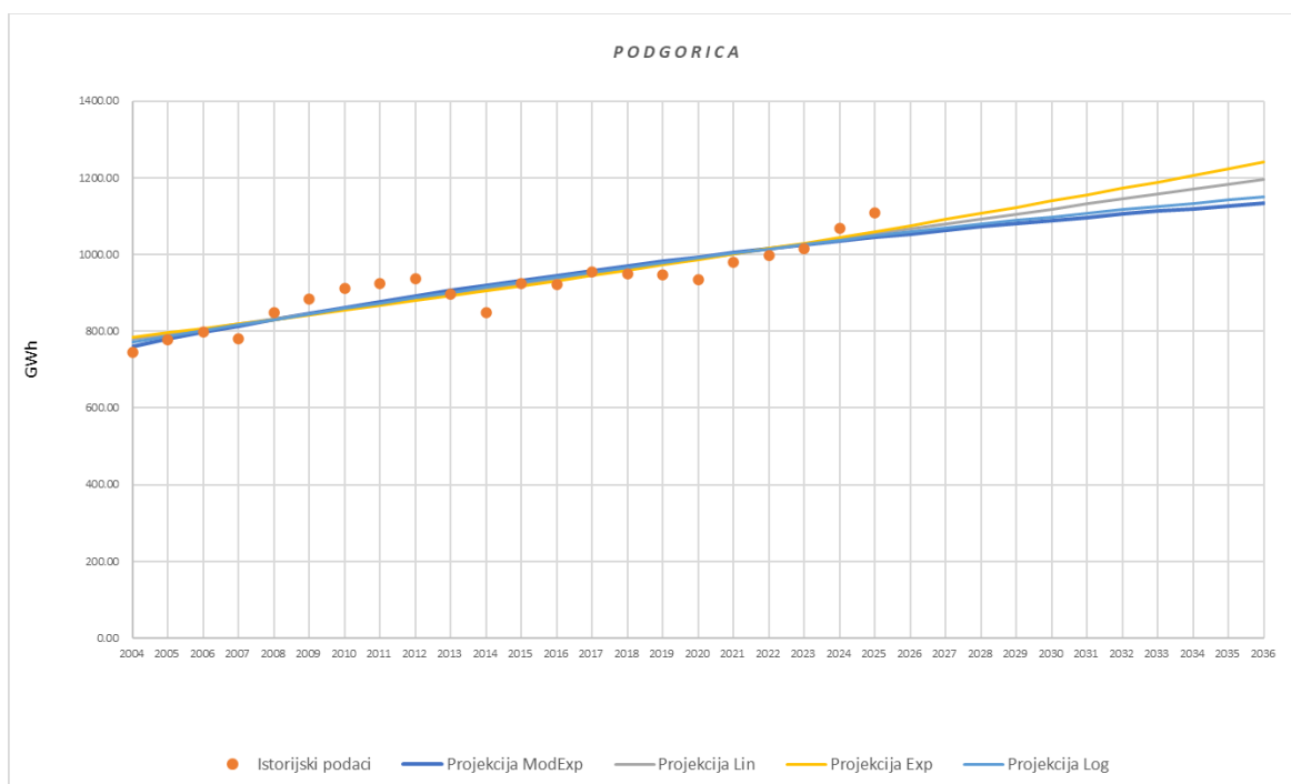
Slika 6-8. Grafički prikaz rezultata prognoznih modela za ED pogon Podgorica
