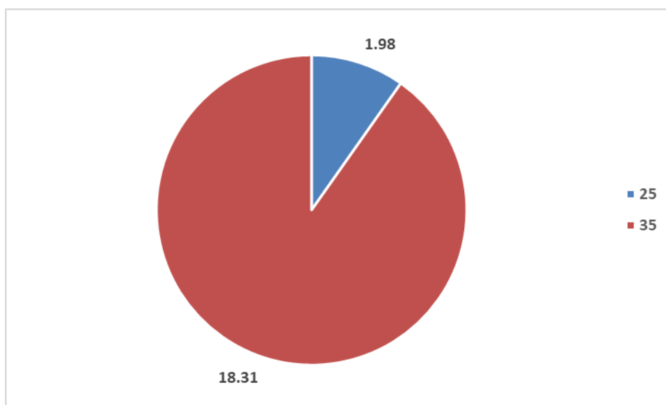
Slika 4-8 Struktura 10 kV nadzemnih vodova od bakra [km]
