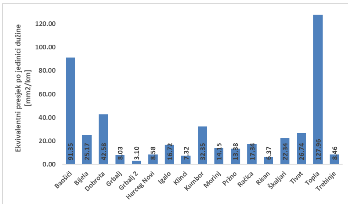
Slika 4-41 Ekvivalentni presjek po jedinici dužine (odnos ekvivalentnog presjeka i ekvivalentne dužine) 10 kV voda po napojnim TS Regiona 5
