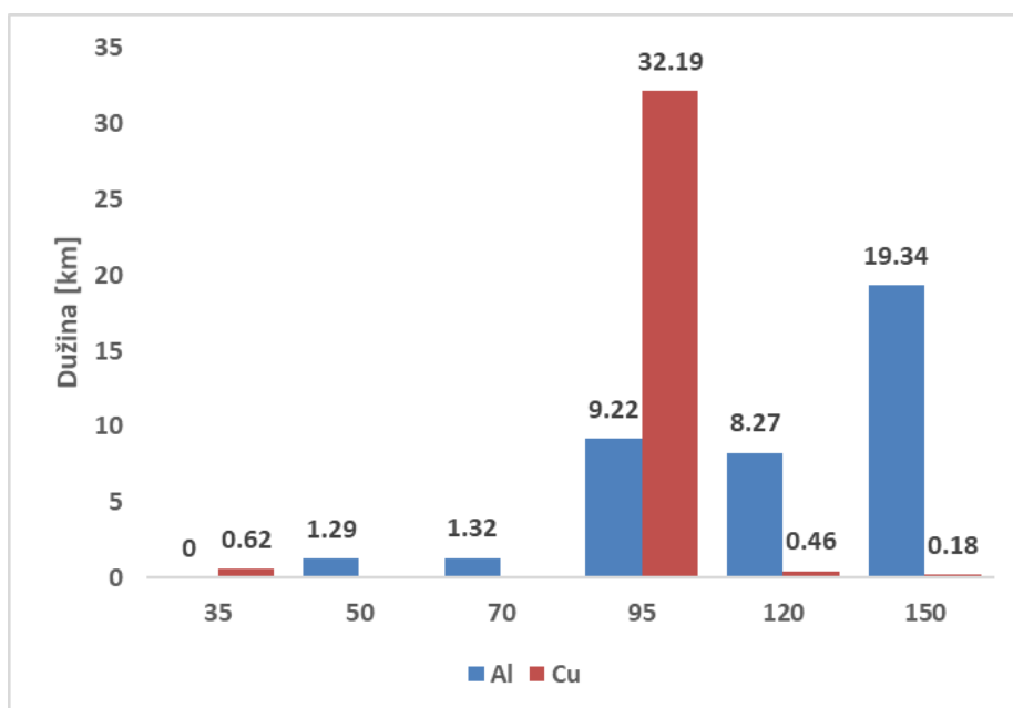
Slika 4-50 Struktura 10 kV kablovske mreže Regiona 7 prema presjecima [km]
