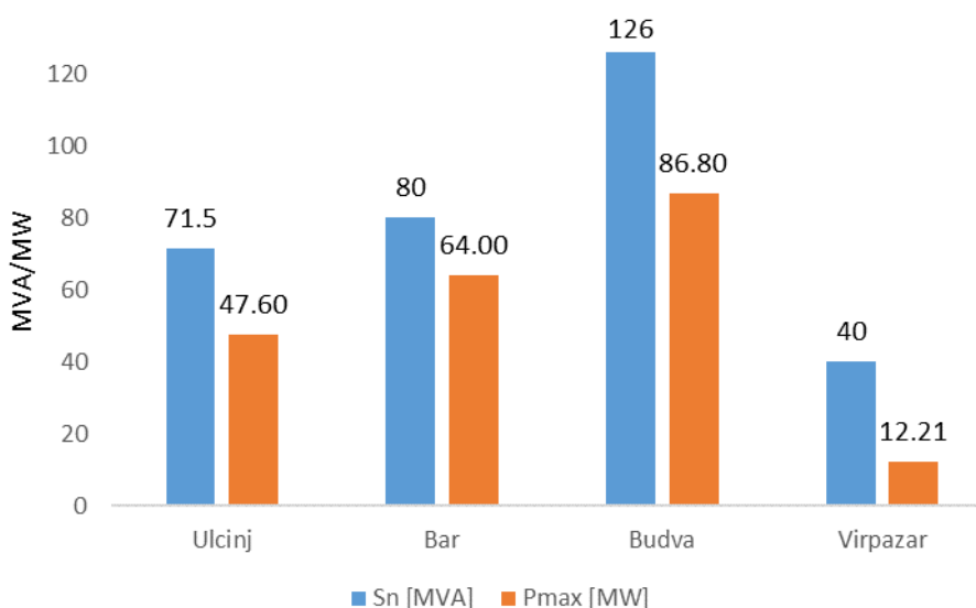
Slika 3-22 Maksimalna opterećenja primarnih TS Regiona 4
