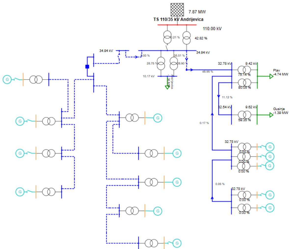
Slika 3-20 Pregled opterećenosti elemenata 35 kV mreže u režimu maksimalnog opterećenja regiona 3 (konzum TS 110/35 kV Andrijevia bez mHE)
