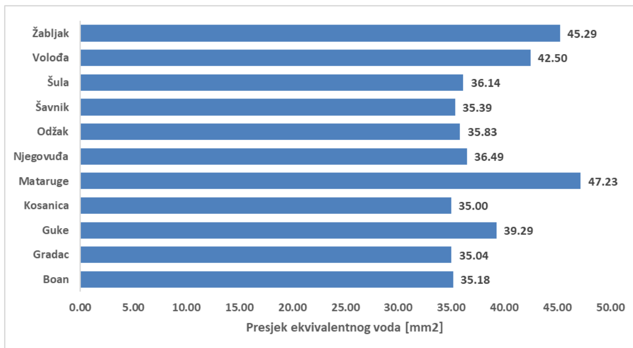
Slika 4-51 Presjek ekvivalentnog 10 kV voda po napojnim TS Regiona 7
