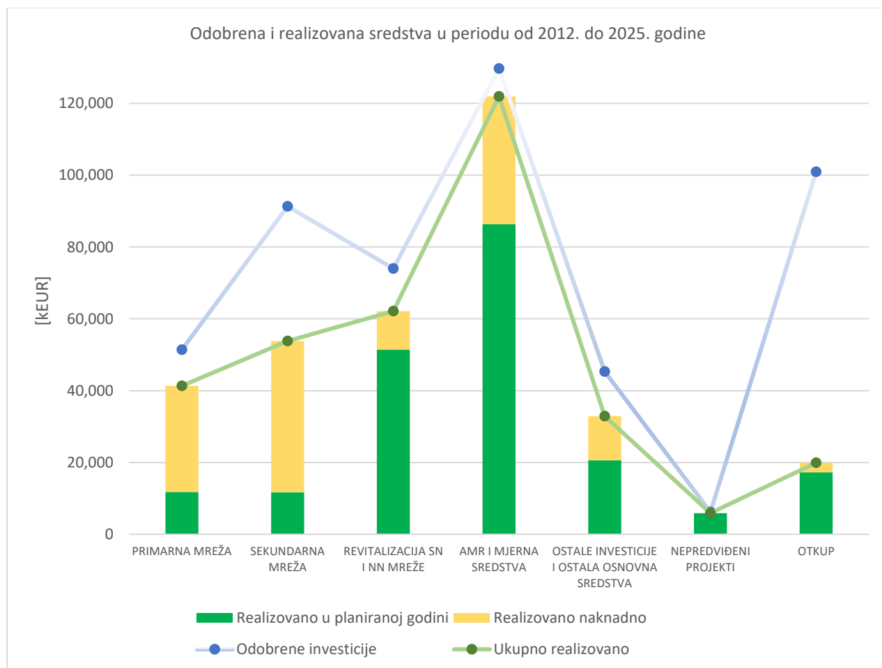
Slika 2-5 Sredstva uložena prema planiranoj dinamici i naknadno realizovana sredstva po kategorijama
