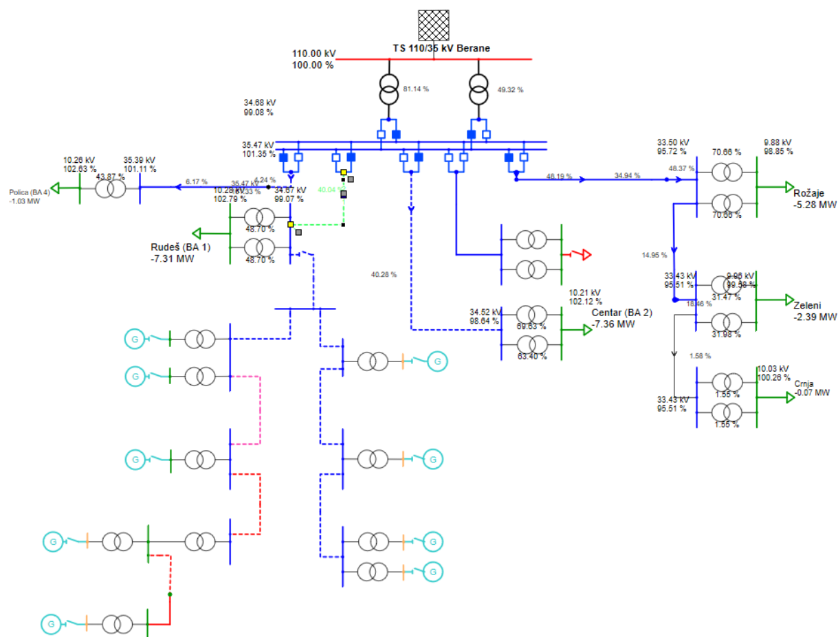
Slika 3-18 Pregled opterećenosti elemenata 35 kV mreže u režimu maksimalnog opterećenja Regiona 3 (konzum TS 110/35 kV Berane bez mHE)
