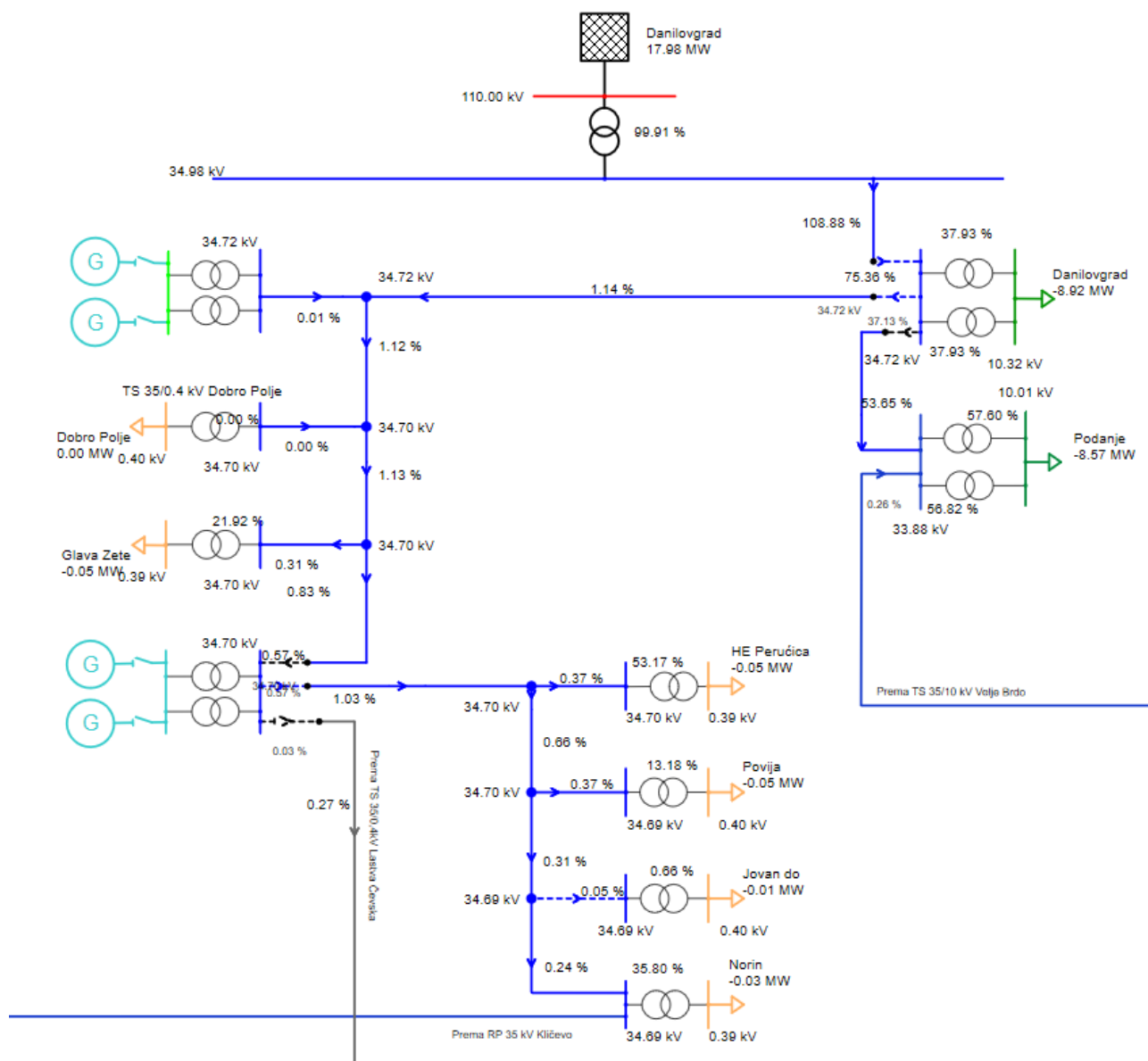
Slika 3-14 Pregled opterećenosti elemenata 35 kV mreže u režimu maksimalnog opterećenja Regiona 2 (konzum TS 110/35 kV Danilovgrad)
