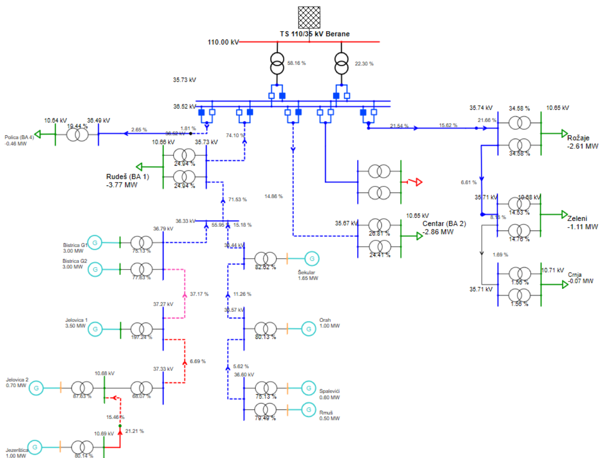
Slika 3-19 Pregled opterećenosti elemenata 35 kV mreže u režimu srednjeg opterećenja Regiona 3 (konzum 110/35 kV Berane sa radom mHE)
