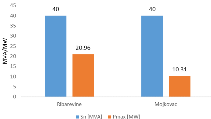
Slika 3-36 Maksimalna opterećenja primarnih TS Regiona 6
