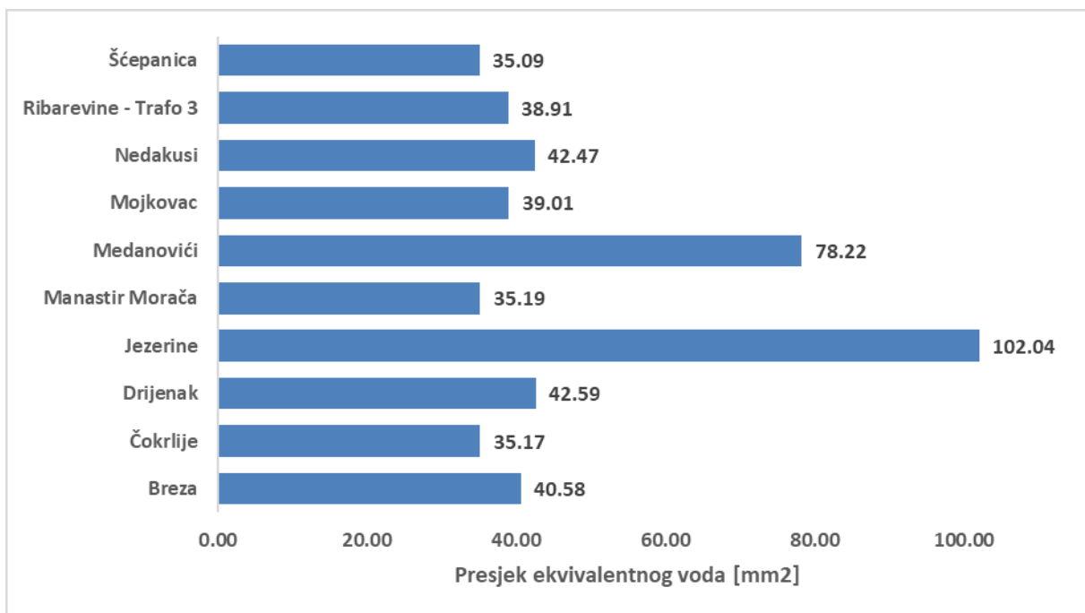
Slika 4-45 Presjek ekvivalentnog 10 kV voda po napojnim TS Regiona 6
