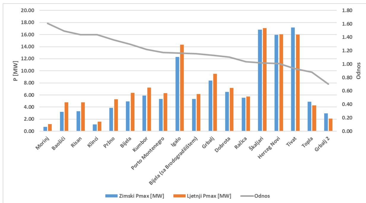
Slika 3-32 Sezonski maksimumi u Regionu 5
