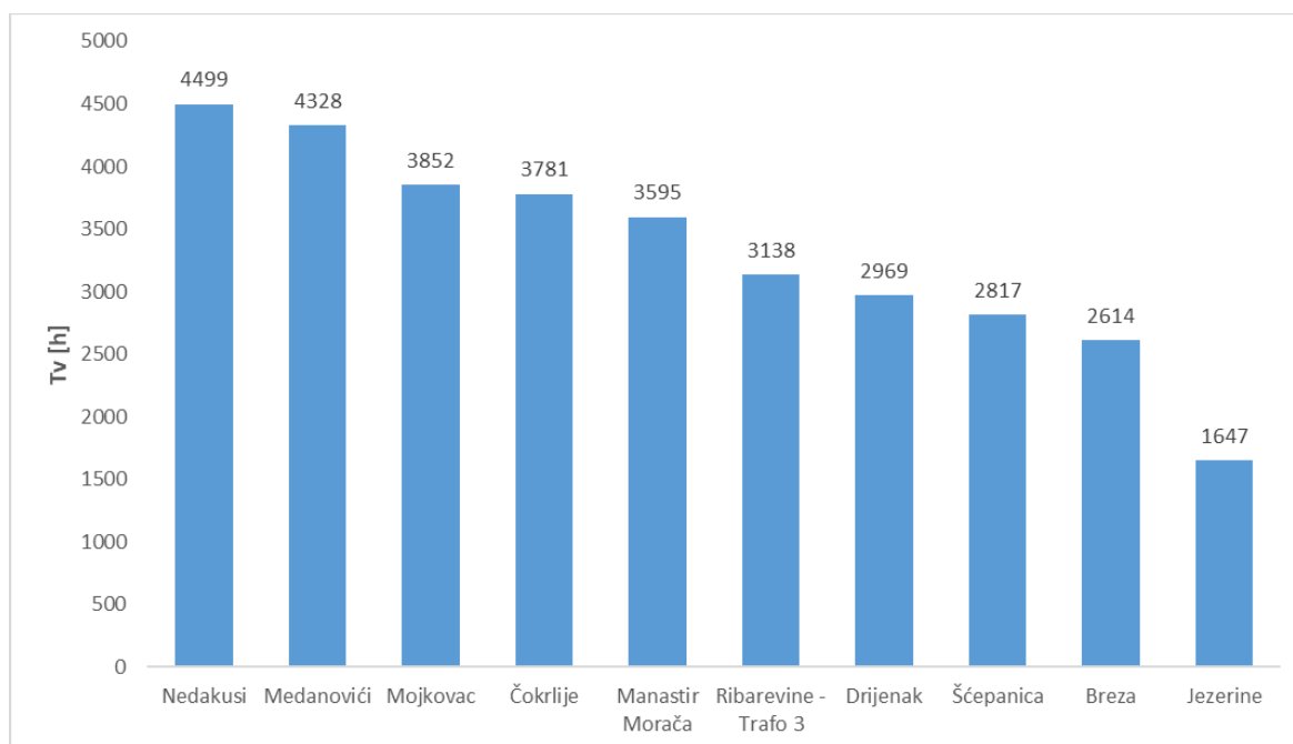
Slika 3-38 Ekvivalentno trajanje vršnog opterećenja sekundarnih TS Regiona 6
