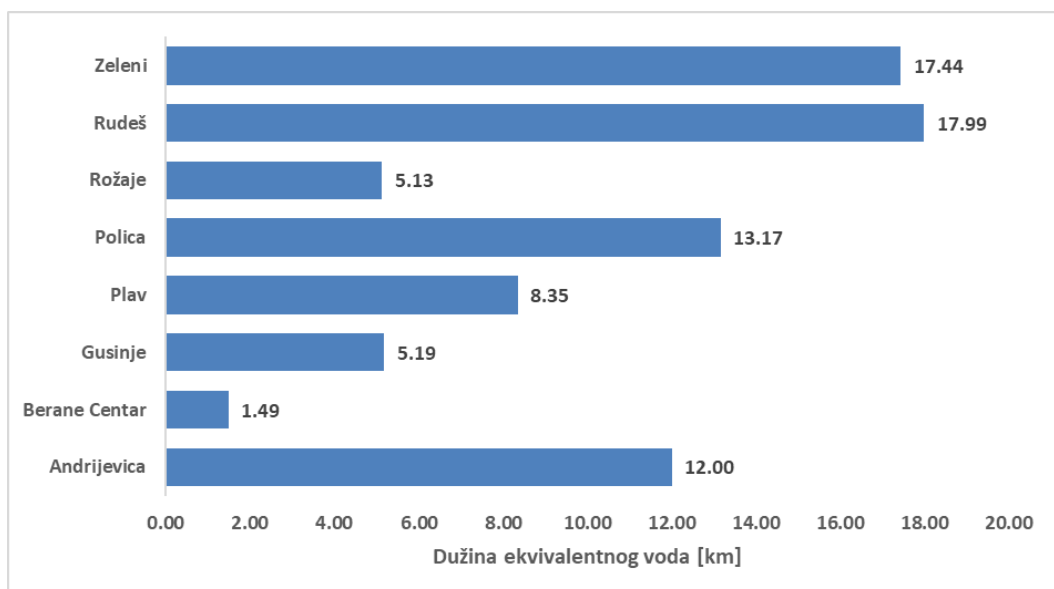
Slika 4-28 Dužina ekvivalentnog 10 kV voda po napojnim TS Regiona 3
