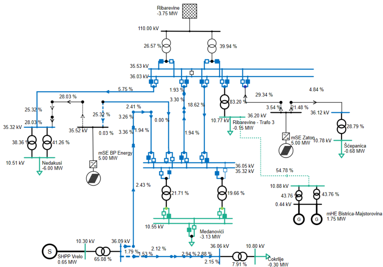
Slika 3-40 Pregled opterećenosti elemenata 35 kV mreže u režimu srednjeg opterećenja Regiona 6 i maksimalne proizvodnje distribuiranih izvora (konzum TS 110/35 kV Ribarevine)
