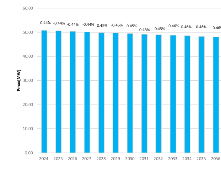
Slika 6-4. Prognoza vršnog opterećenja Regiona 1 za period 2024 – 2036. godine
