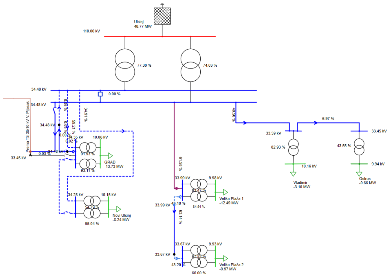
Slika 3-26 Pregled opterećenosti elemenata 35 kV mreže u režimu maksimalnog opterećenja Regiona 4 (konzum TS 110/35 kV Ulcinj)
