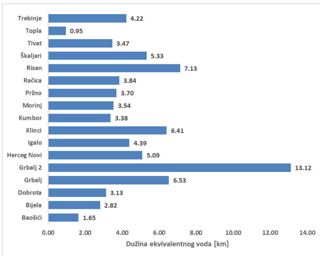
Slika 4-40 Dužina ekvivalentnog 10 kV voda po napojnim TS Regiona 5
