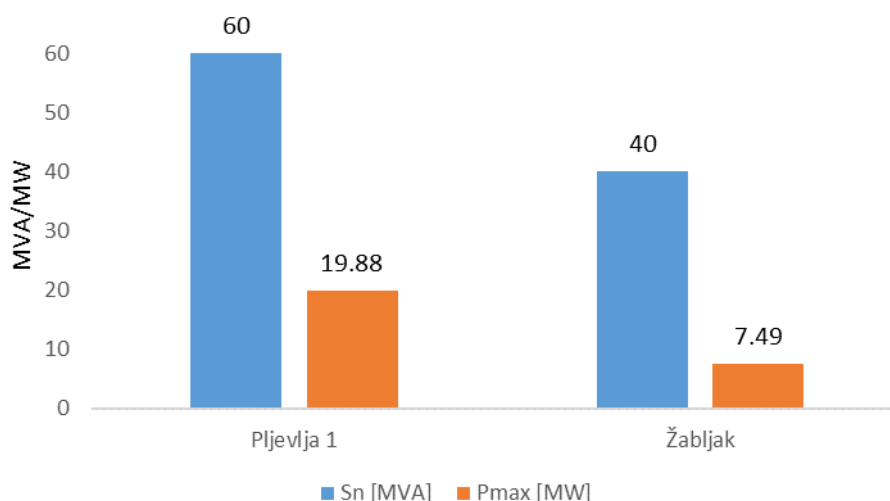
Slika 3-42 Maksimalna opterećenja primarnih TS Regiona 7
