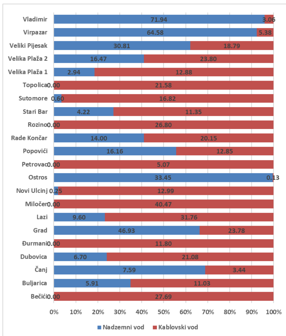
Slika 4-30 Učešće nadzemne i kablovske 10 kV mreže po napojnim TS Regiona 4
