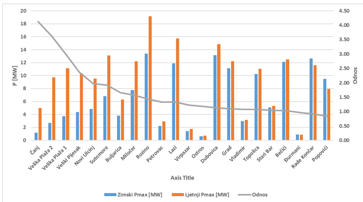
Slika 3-24 Sezonski maksimumi u Regionu 4
