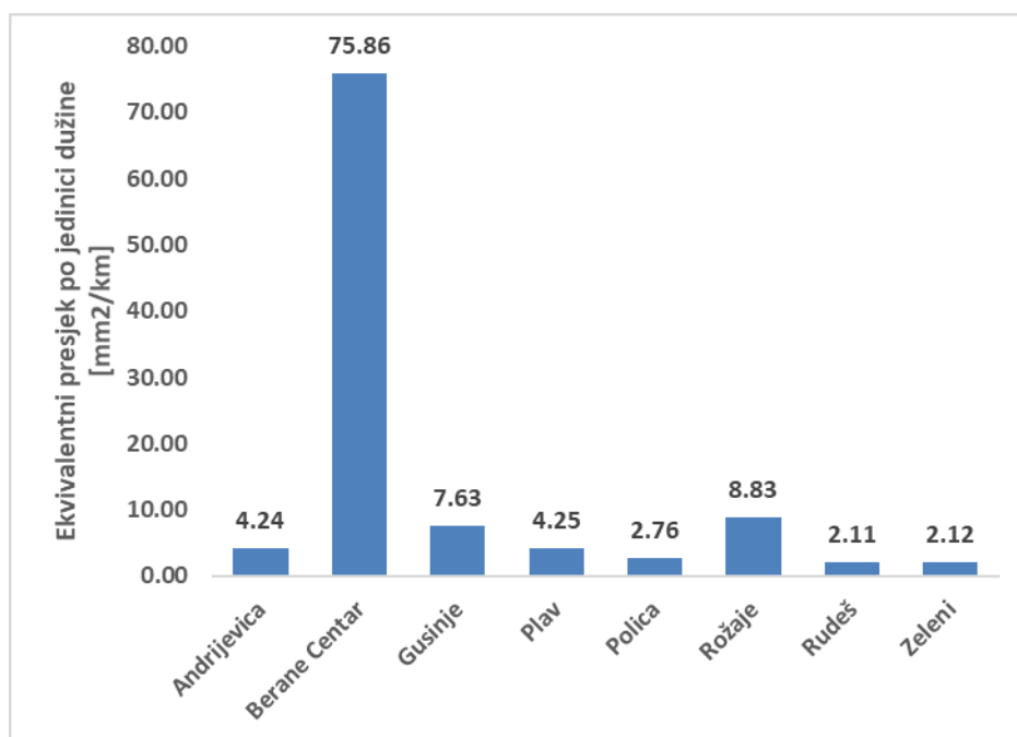
Slika 4-29 Ekvivalentni presjek po jedinici dužine (odnos ekvivalentnog presjeka i ekvivalentne dužine) 10 kV voda po napojnim TS Regiona 3
