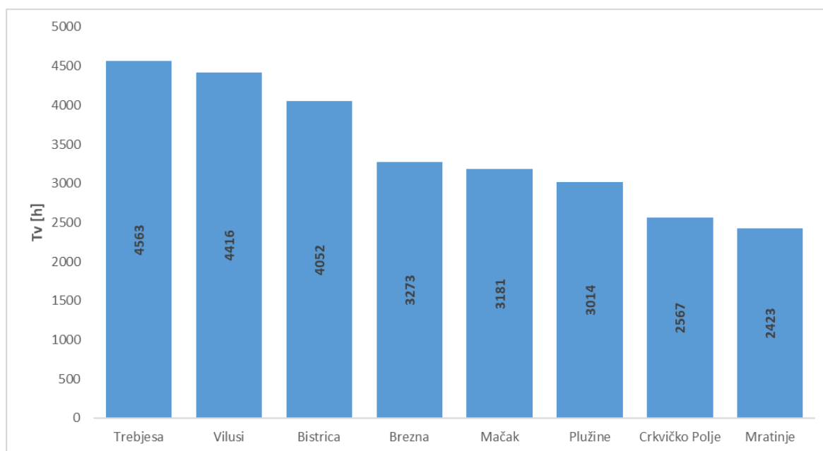
Slika 3-6 Ekvivalentno trajanje vršnog opterećenja sekundarnih TS Regiona 1
