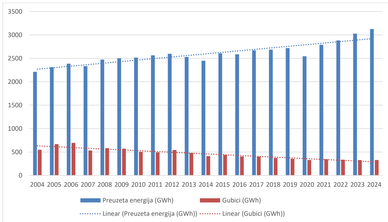
Slika 2-12 Preuzete i energije gubitaka u GWh
