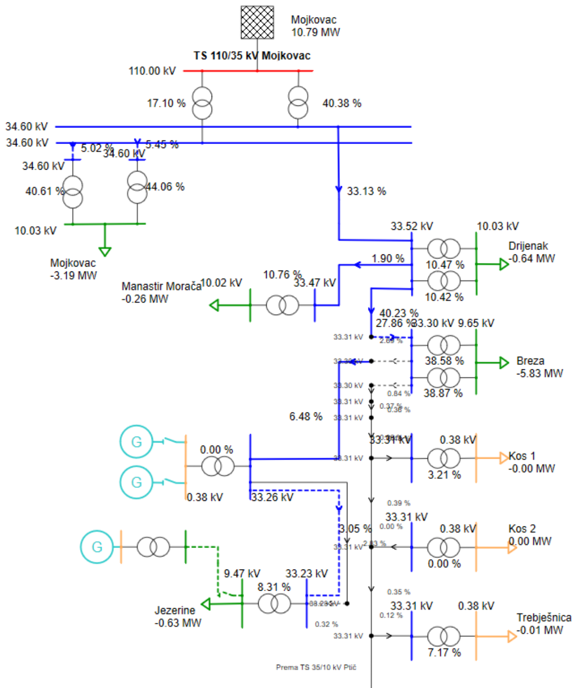
Slika 3-41 Pregled opterećenosti elemenata 35 kV mreže u režimu maksimalnog opterećenja Regiona 6 (Konzum TS 110/35 kV Mojkovac)
