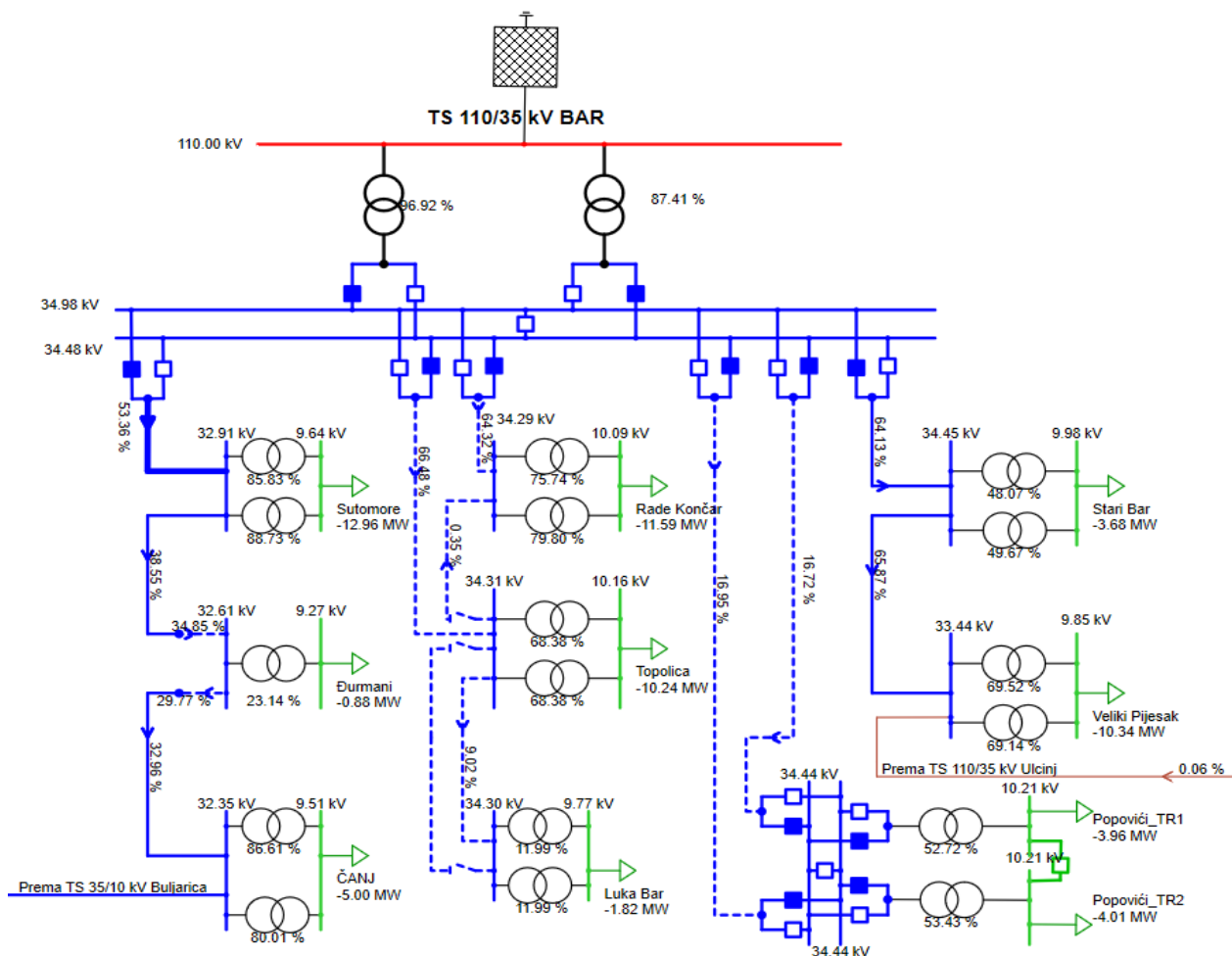
Slika 3-27 Pregled opterećenosti elemenata 35 kV mreže u režimu maksimalnog opterećenja Regiona 4 (konzum TS 110/35 kV Bar)
