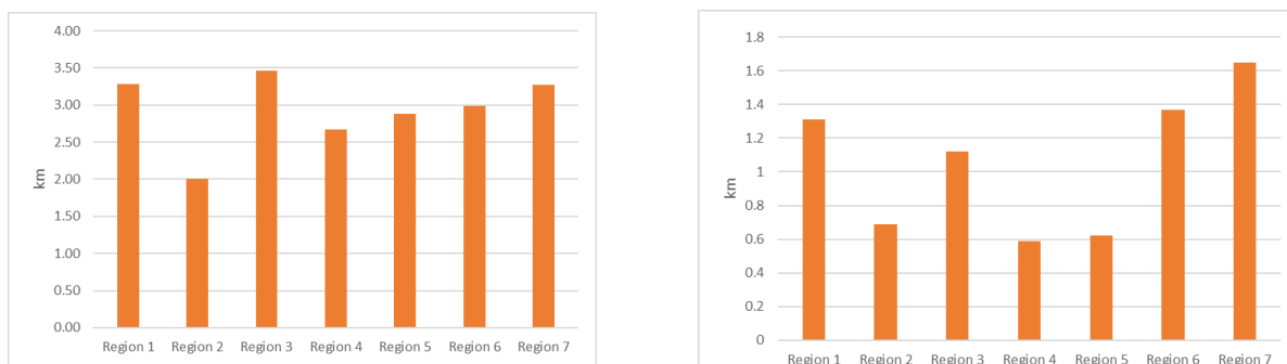
Slika 5-3 Dužina NN mreže po transformatoru X/0,4 kV (a) i po izvodu TS X/0,4 kV (b) po regionima
