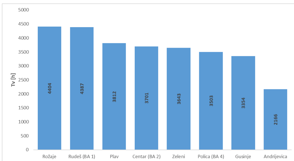
Slika 3-17 Ekvivalentno trajanje vršnog opterećenja sekundarnih TS Regiona 3
