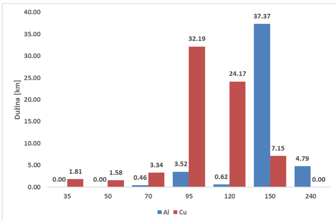
Slika 4-44 Struktura 10 kV kablovske mreže Regiona 6 prema presjecima [km]
