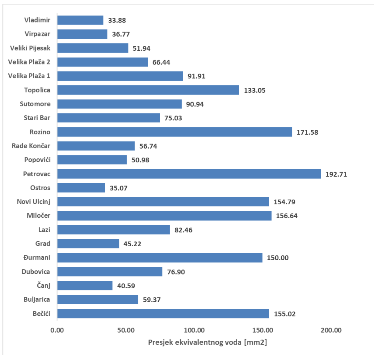
Slika 4-33 Presjek ekvivalentnog 10 kV voda po napojnim TS Regiona 4
