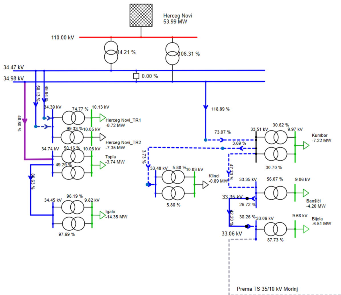
Slika 3-34 Pregled opterećenosti elemenata 35 kV mreže u režimu maksimalnog opterećenja Regiona 5 (konzum TS 110/35 kV Herceg Novi)
