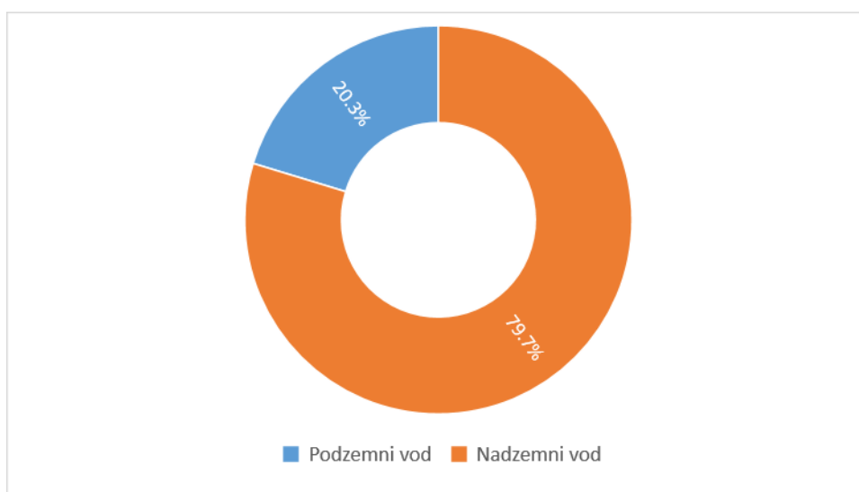
Slika 5-1 Struktura niskonaponske mreže ED Crne Gore prema tipu
