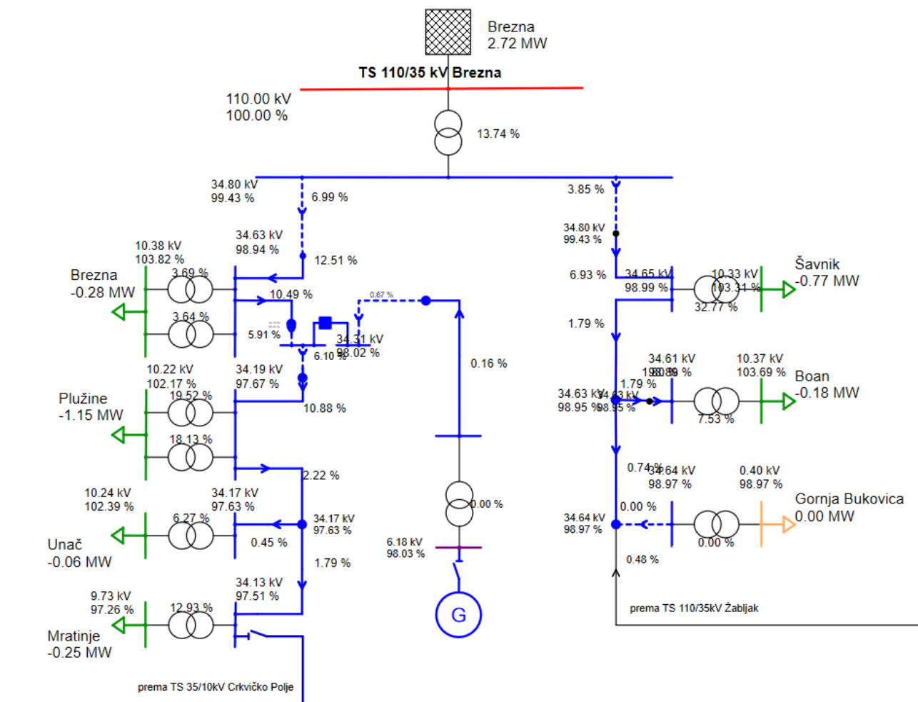
Slika 3-8 Pregled opterećenosti elemenata 35 kV mreže u režimu maksimalnog opterećenja (drugi dio)
