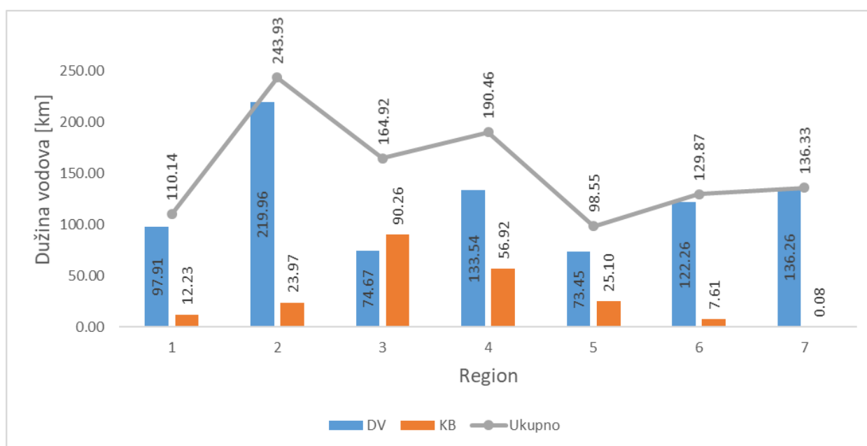
Slika 3-3 Struktura tipova vodova po Regionima
