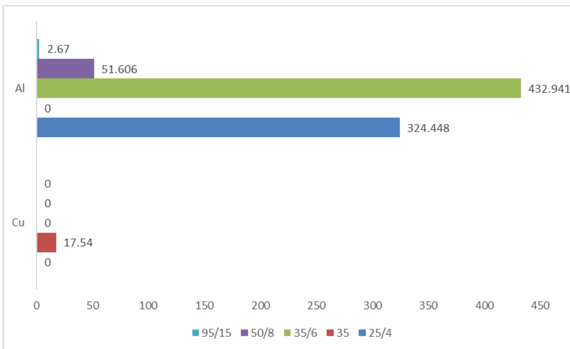
Slika 4-19 Struktura 10 kV nadzemne mreže Regiona 2 prema presjecima [km]
