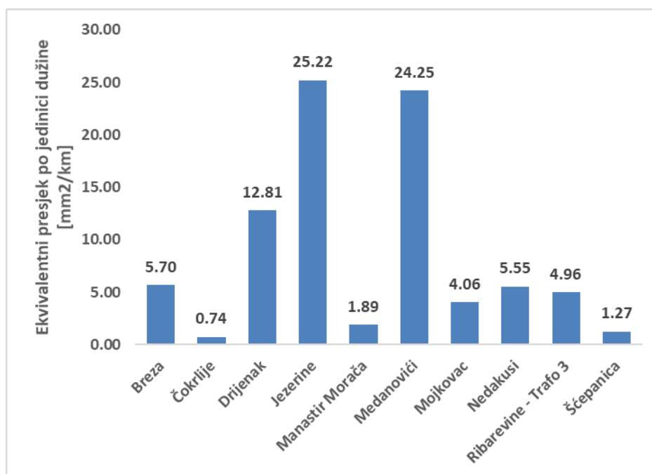
Slika 4-47 Ekvivalentni presjek po jedinici dužine (odnos ekvivalentnog presjeka i ekvivalentne dužine) 10 kV voda po napojnim TS Regiona 6
