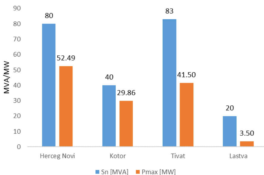
Slika 3-30 Maksimalna opterećenja primarnih TS Regiona 5
