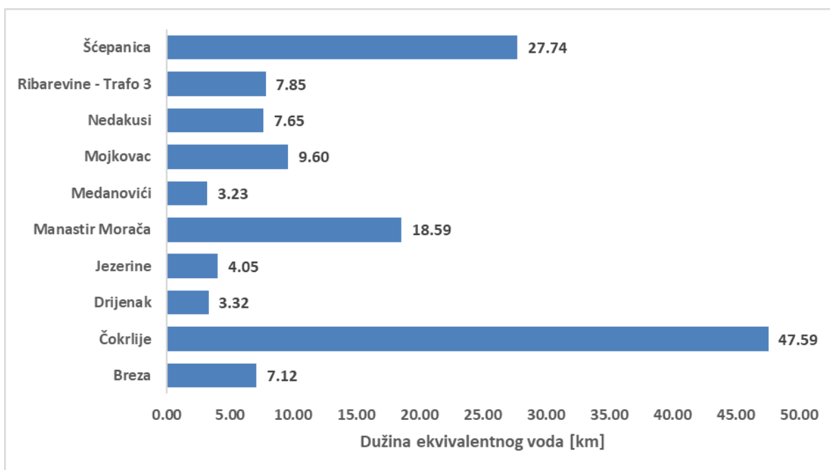
Slika 4-46 Dužina ekvivalentnog 10 kV voda po napojnim TS Regiona 6
