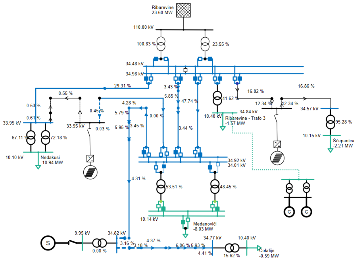
Slika 3-39 Pregled opterećenosti elemenata 35 kV mreže u režimu maksimalnog opterećenja Regiona 6 (konzum TS 110/35 kV Ribarevine )
