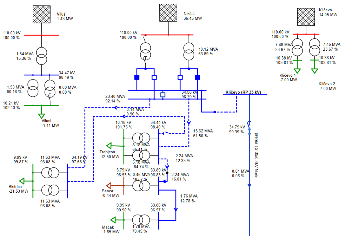
Slika 3-7 Pregled opterećenosti elemenata 35 kV mreže u režimu maksimalnog opterećenja (prvi dio)
