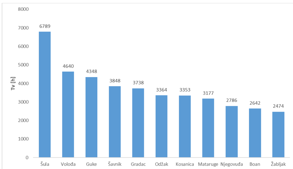
Slika 3-44 Ekvivalentno trajanje vršnog opterećenja sekundarnih TS Regiona 7
