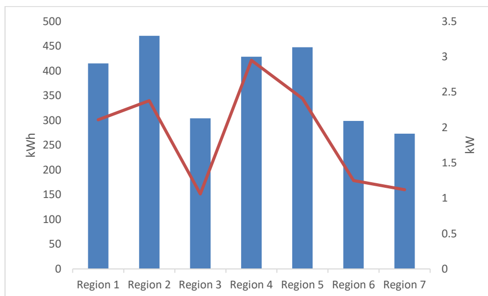
Slika 5-6 Prosječna mjesečna potrošnja el. energije i vršna snaga potrošača po regionima
