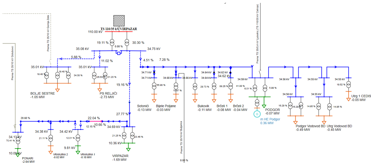
Slika 3-28 Pregled opterećenosti elemenata 35 kV mreže u režimu maksimalnog opterećenja Regiona 4 (drugi diokonzum TS 110/35 kV Virpazar)
