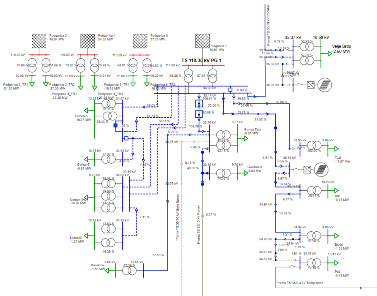
Slika 3-12 Pregled opterećenosti elemenata 35 kV mreže u režimu maksimalnog opterećenja Regiona 2 (konzum TS 110/35 kV Podgorica 1)
