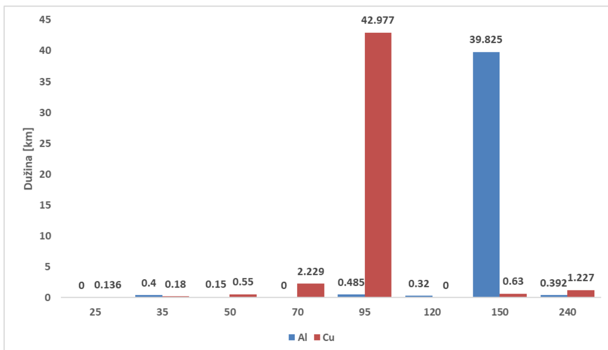
Slika 4-26 Struktura 10 kV kablovske mreže Regiona 3 prema presjecima [km]
