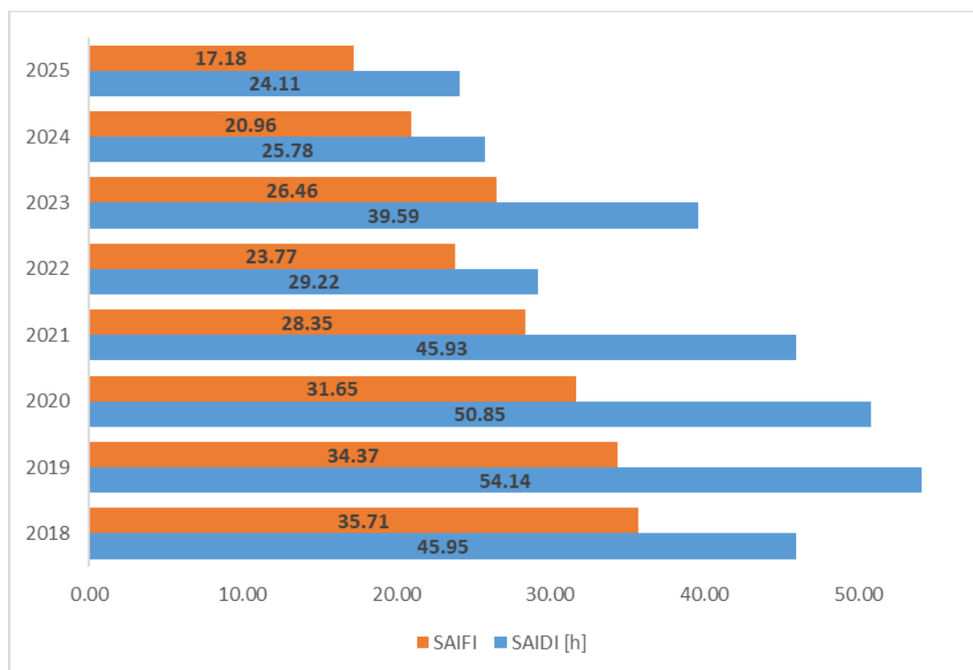
Slika 3-53 Pregled SAIDI i SAIFI po godinama
