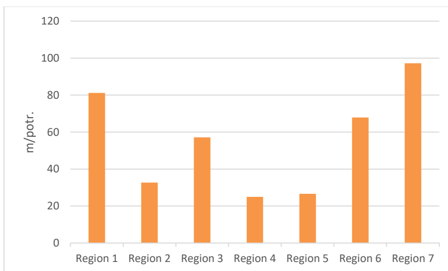
Slika 5-4 Dužina NN mreže po NN potrošaču po regionima
