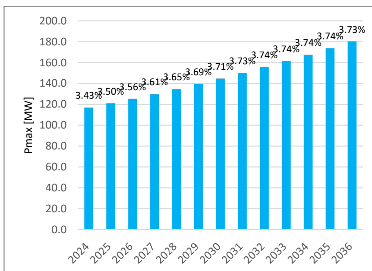
Slika 6-31. Prognoza vršnog opterećenja Regiona 5 za period 2024 – 2036. godina.
