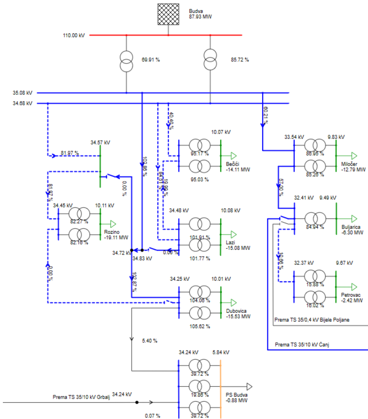
Slika 3-29 Pregled opterećenosti elemenata 35 kV mreže u režimu maksimalnog opterećenja Regiona 4 (drugi diokonzum TS 110/35 kV Budva)
