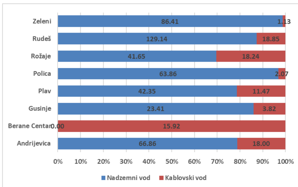
Slika 4-24 Učešće nadzemne i kablovske 10 kV mreže po napojnim TS Regiona 3
