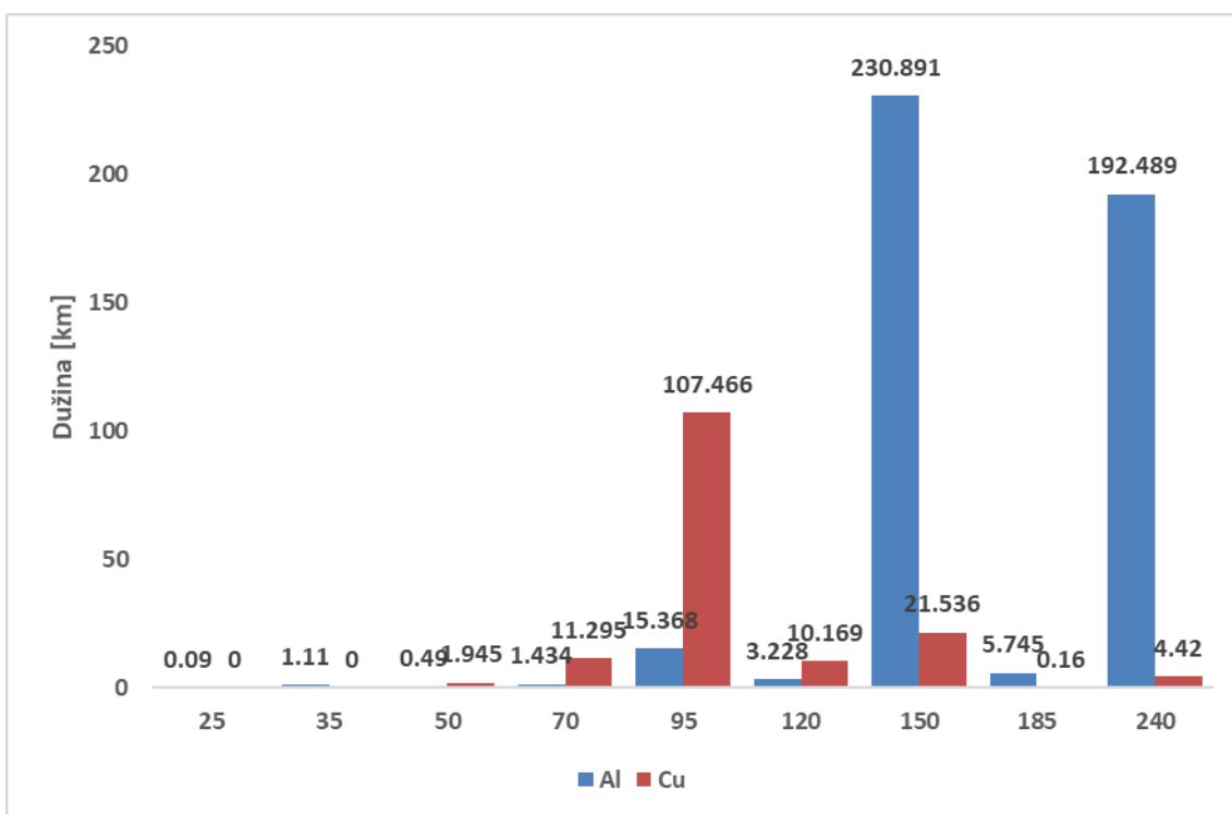
Slika 4-20 Struktura 10 kV kablovske mreže Regiona 2 prema presjecima [km]
