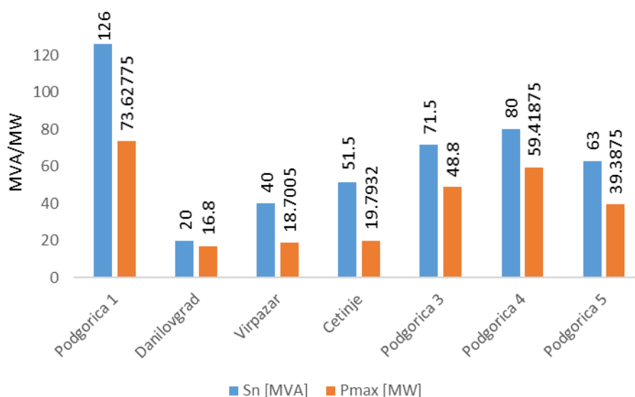
Slika 3-9 Maksimalna opterećenja primarnih TS Regiona 2
