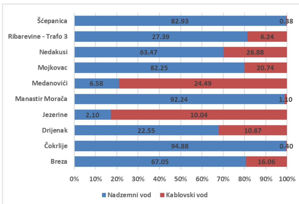
Slika 4-42 Učešće nadzemne i kablovske 10 kV mreže po napojnim TS Regiona 6
