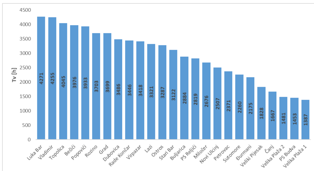
Slika 3-25 Ekvivalentno trajanje vršnog opterećenja sekundarnih TS Regiona 4
