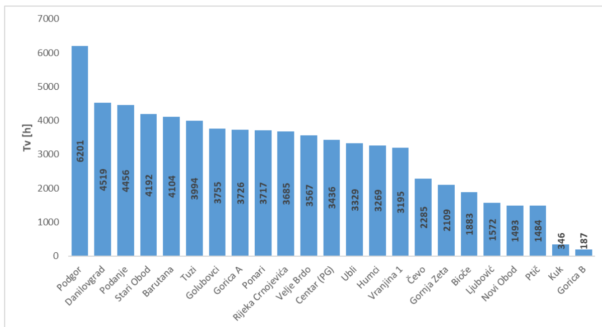
Slika 3-11 Ekvivalentno trajanje vršnog opterećenja sekundarnih TS Regiona 2
