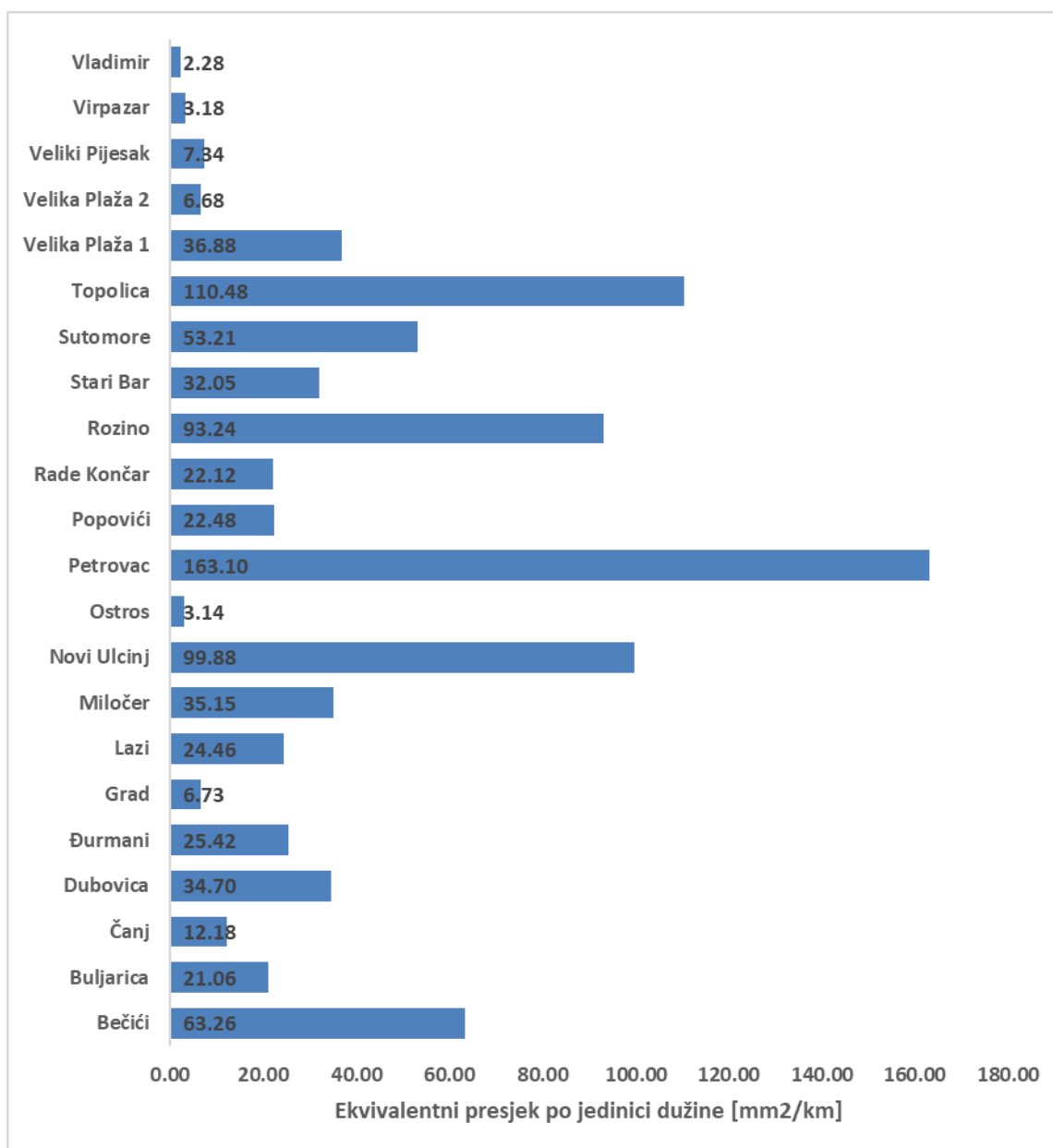
Slika 4-35 Ekvivalentni presjek po jedinici dužine (odnos ekvivalentnog presjeka i ekvivalentne dužine) 10 kV voda po napojnim TS Regiona 4
