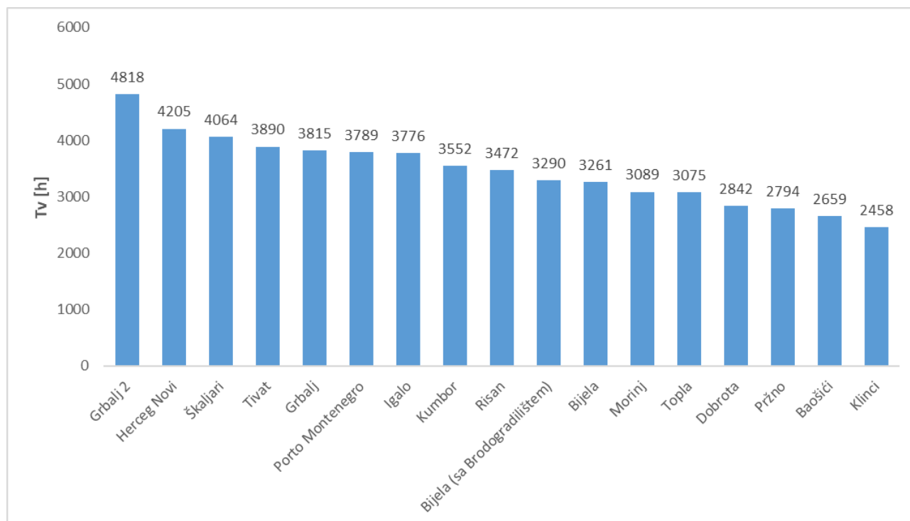
Slika 3-33 Ekvivalentno trajanje vršnog opterećenja sekundarnih TS Regiona 5
