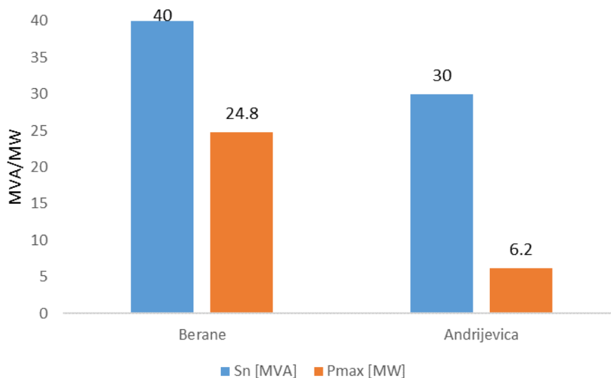
Slika 3-15 Maksimalna opterećenja primarnih TS Regiona 3
