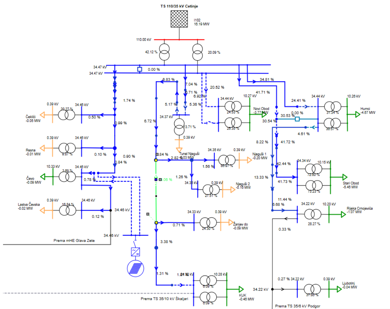
Slika 3-13 Pregled opterećenosti elemenata 35 kV mreže u režimu maksimalnog opterećenja Regiona 2 (konzum TS 110/35 kV Cetinje)
